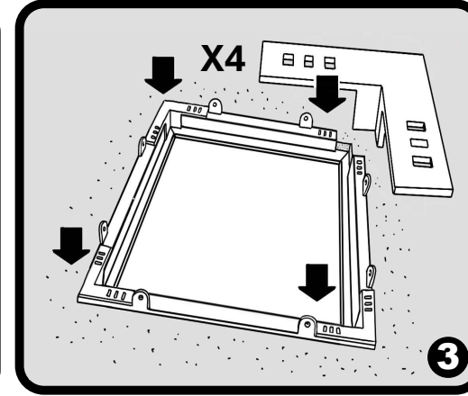
התקנת 4 פינות חיבור
