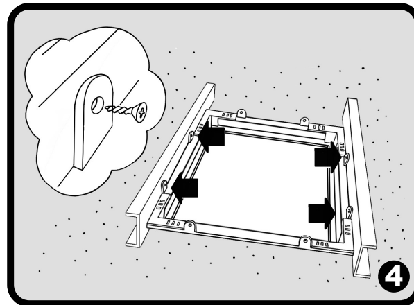
אופציה של תוספת קורות חיזוק וחיבור אל המסגרת בברגים לפי דרישת מתכנן
