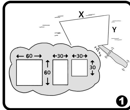
חיתוך תקרת גבס לפי מידות
